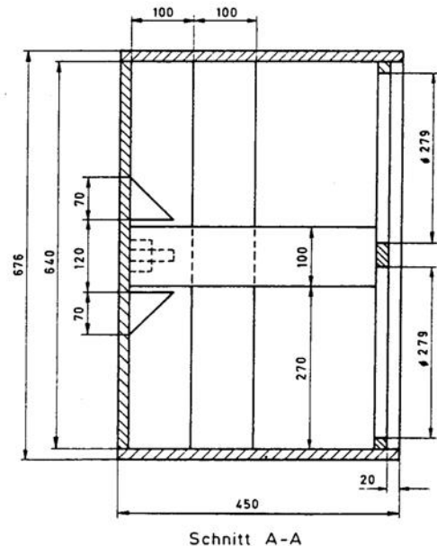
Schnitt A-A
